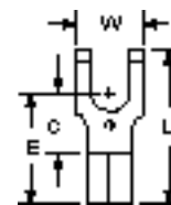
MU10-10FFB Stud Size 10 Wire Range 12-10
